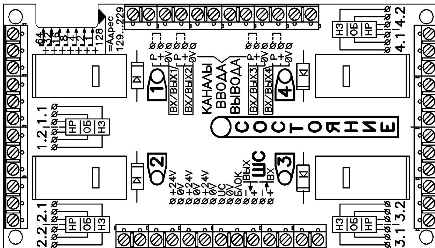
Внешний вид и расположение клемм БВВ-А-01
