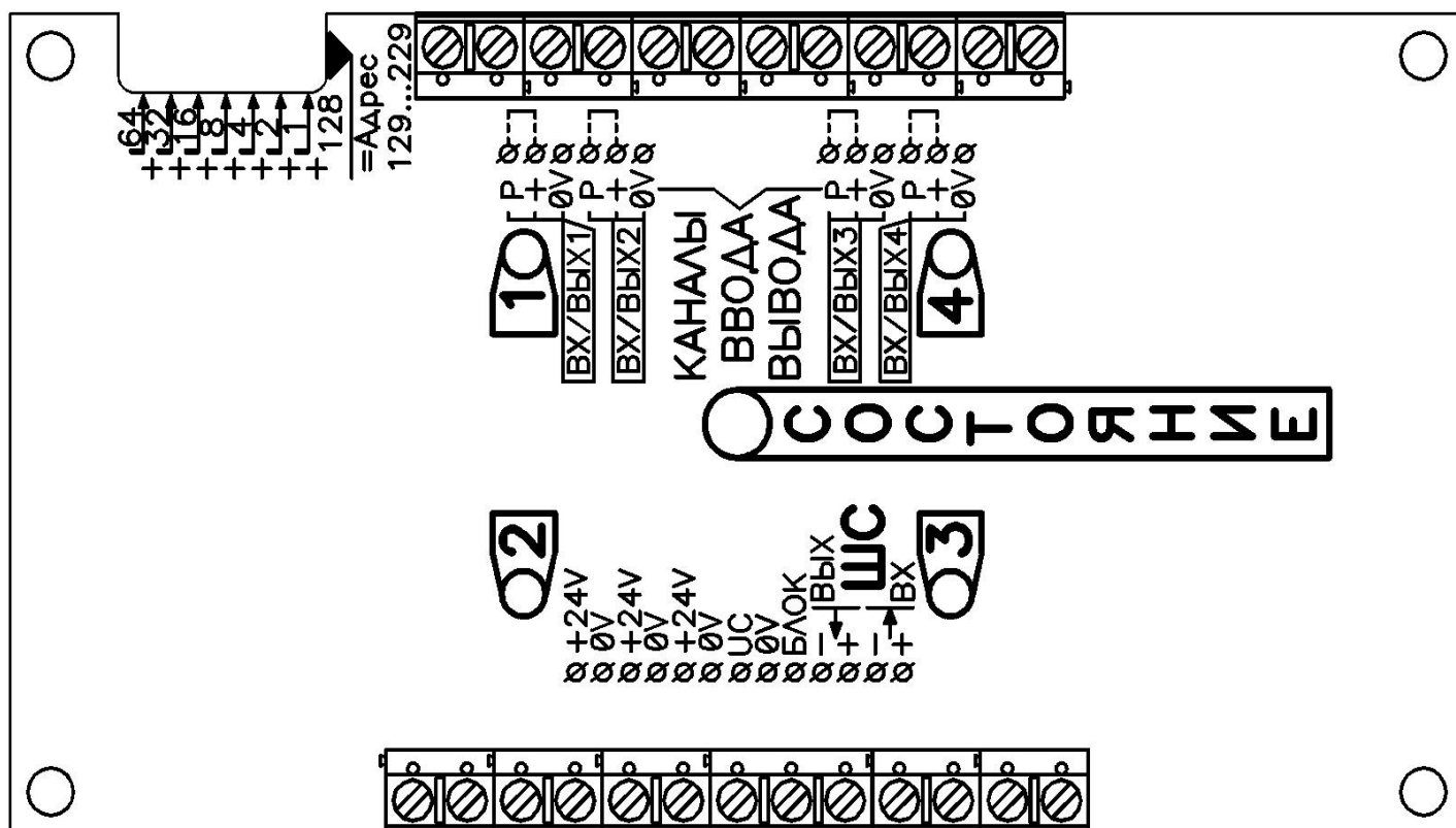
Внешний вид и расположение клемм БВВ-А, БВВ-А-02
